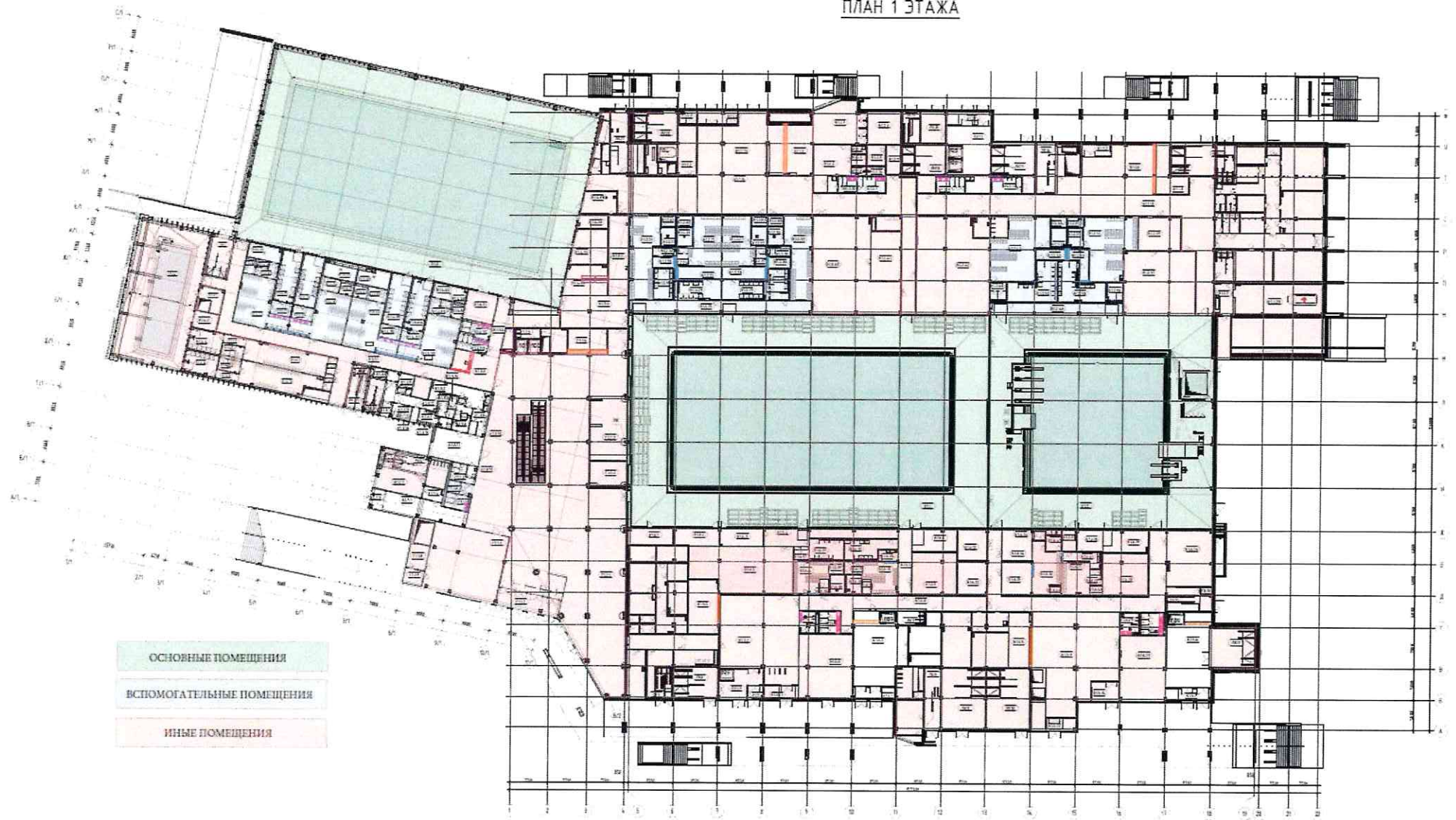
ПЛАН 1 ЭТАЖА
